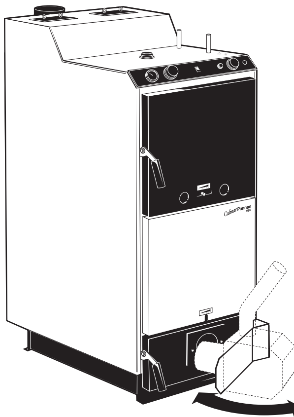
7.2 Principinstallation av oljebrännare monterad med svängarm 611 5378 (Tillbehör)
